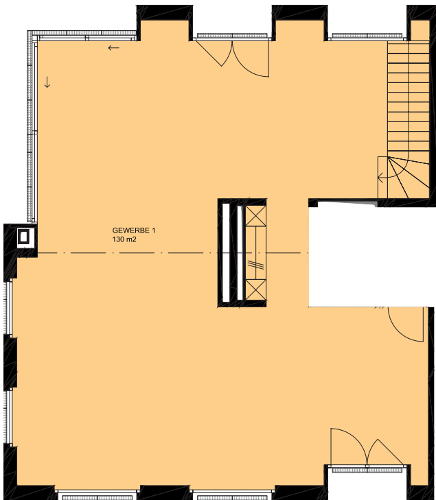
Erdgeschoss
